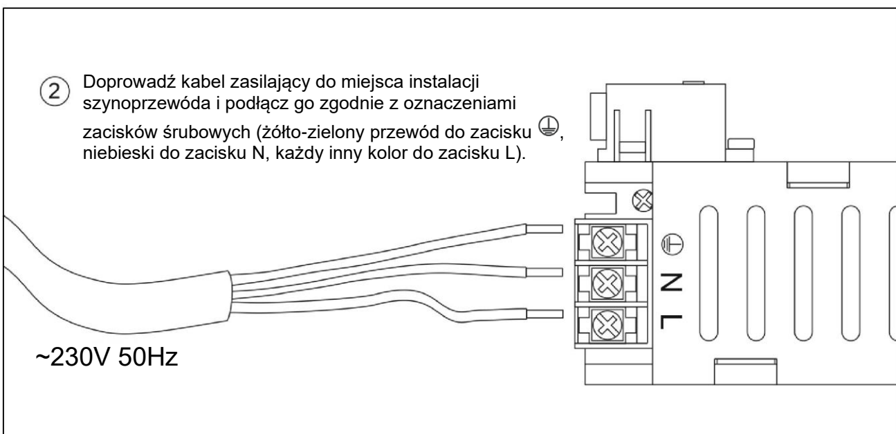
Rys. 2 Podłączenie kabla zasilającego
