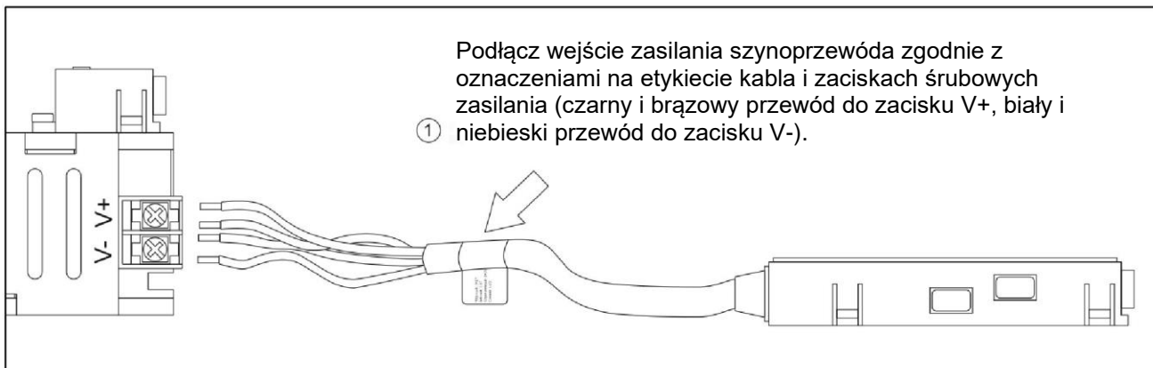
Rys. 1 Podłączenie wejścia zasilania szynoprzewodu
